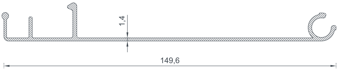
6161 BİRİM AĞIRLIK - Weight 1,622 (kg/mt)
