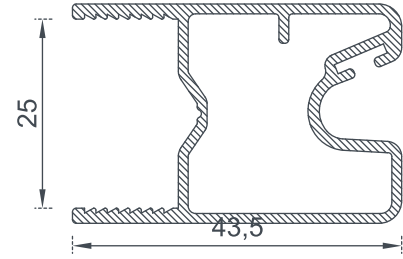
6170 BİRİM AĞIRLIK - Weight 1,622 (kg/mt)
