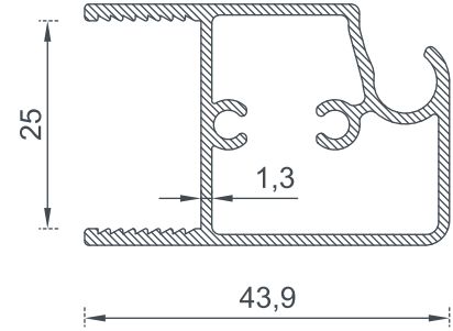
6164 BİRİM AĞIRLIK - Weight 1,622 (kg/mt)
