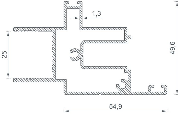
6165 BİRİM AĞIRLIK - Weight 1,622 (kg/mt)
