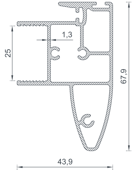
6171 BİRİM AĞIRLIK - Weight 1,622 (kg/mt)
