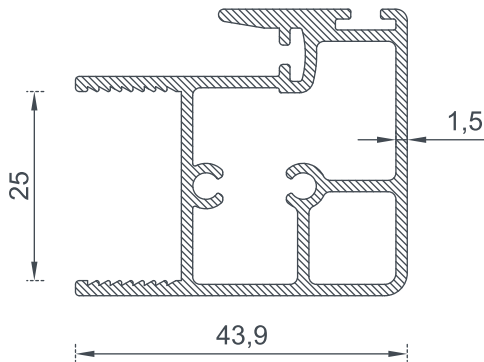
6167 BİRİM AĞIRLIK - Weight 1,622 (kg/mt)
