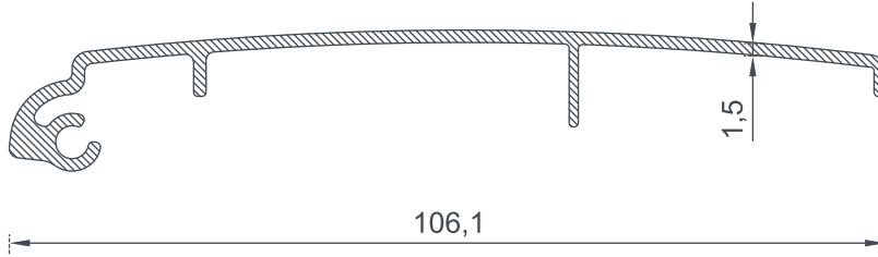
6163 BİRİM AĞIRLIK - Weight 1,622 (kg/mt)
