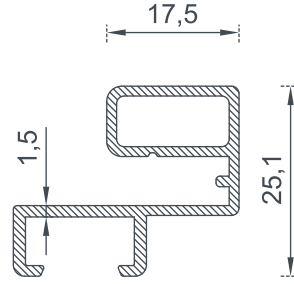
6162 BİRİM AĞIRLIK - Weight 1,622 (kg/mt)
