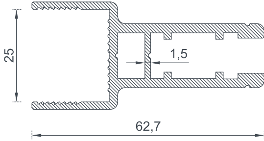
6166 BİRİM AĞIRLIK - Weight 1,622 (kg/mt)
