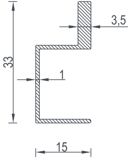
7010 BİRİM AĞIRLIK - Weight 0,246 (kg/mt)
