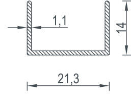
7012 BİRİM AĞIRLIK - Weight 0,140 (kg/mt)
