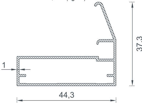
3929 BİRİM AĞIRLIK - Weight 0,426 (kg/mt)
