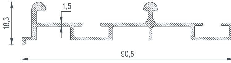
1211 BİRİM AĞIRLIK - Weight 0,734 (kg/mt)
