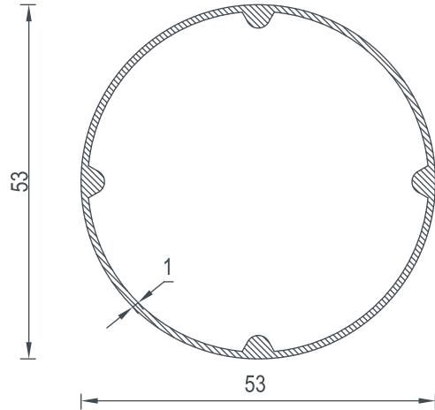
2572 BİRİM AĞIRLIK - Weight 0,533 (kg/mt)
