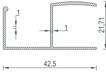
7014 BİRİM AĞIRLIK - Weight 0,293 (kg/mt)
