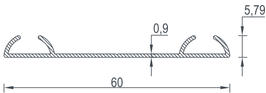
1206 BİRİM AĞIRLIK - Weight 0,212 (kg/mt)
