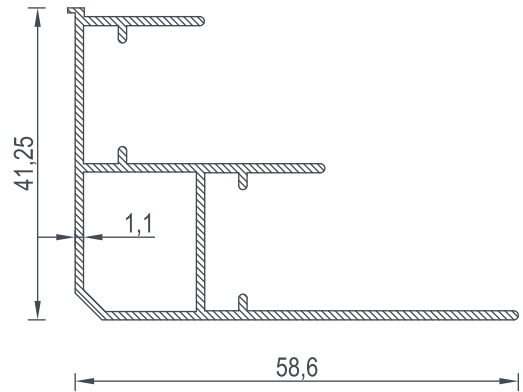
1209 BİRİM AĞIRLIK - Weight 0,532 (kg/mt)
