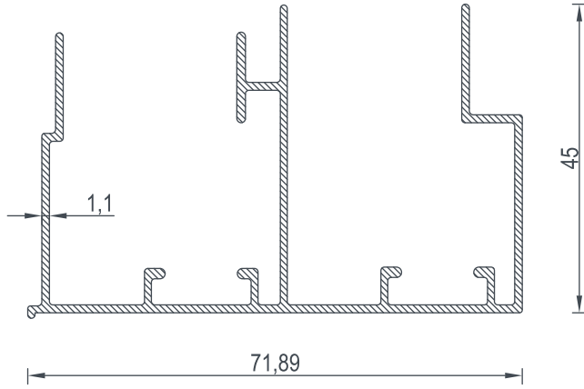
1214 BİRİM AĞIRLIK - Weight 0,772 (kg/mt)
