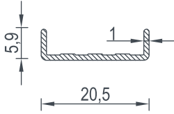
7013 BİRİM AĞIRLIK - Weight 0,085 (kg/mt)
