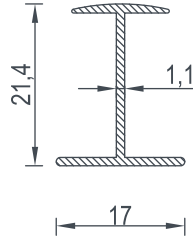
7011 BİRİM AĞIRLIK - Weight 0,140 (kg/mt)
