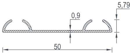
1204 BİRİM AĞIRLIK - Weight 0,188 (kg/mt)
