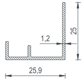
1228 BİRİM AĞIRLIK - Weight 0,200 (kg/mt)
