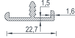
1202 BİRİM AĞIRLIK - Weight 0,160 (kg/mt)
