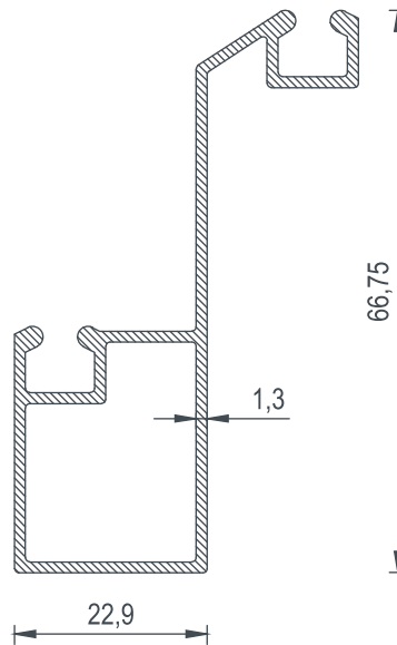
1230 BİRİM AĞIRLIK - Weight 0,656 (kg/mt)
