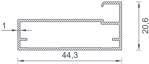
3928 BİRİM AĞIRLIK - Weight 0,371 (kg/mt)
