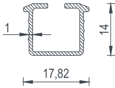
1223 BİRİM AĞIRLIK - Weight 0,149 (kg/mt)
