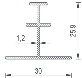
1229 BİRİM AĞIRLIK - Weight 0,232 (kg/mt)
