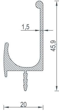
7015 BİRİM AĞIRLIK - Weight 0,429 (kg/mt)
