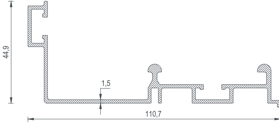
1203 BİRİM AĞIRLIK - Weight 1,018 (kg/mt)
