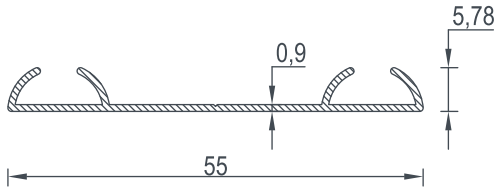
1205 BİRİM AĞIRLIK - Weight 0,193 (kg/mt)
