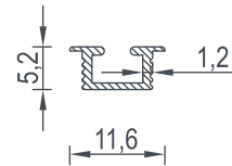
1208 BİRİM AĞIRLIK - Weight 0,056 (kg/mt)
